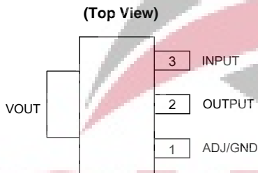
SOT223/ H Package
